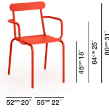
DINING ARMCHAIR / SILLA CON BRAZOS
