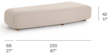
SOFA SEAT 01 / ASIENTO 01
